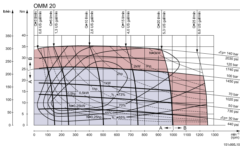
OMM 20 function diagram
