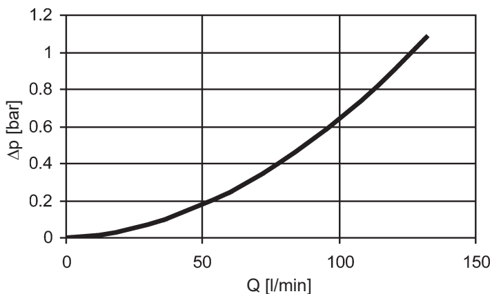
DFF 60, 110, 140
