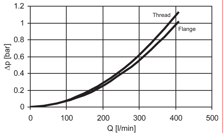
DFF 160, 240, 280
