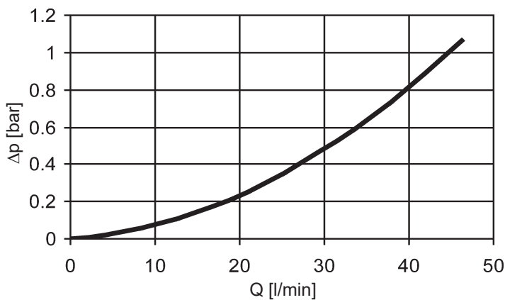
DF 60, 110, 140
