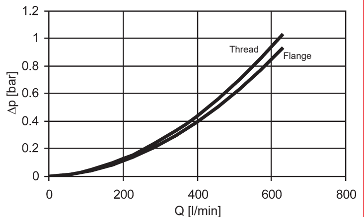
DFF 330, 500, 660, 990, 1320
