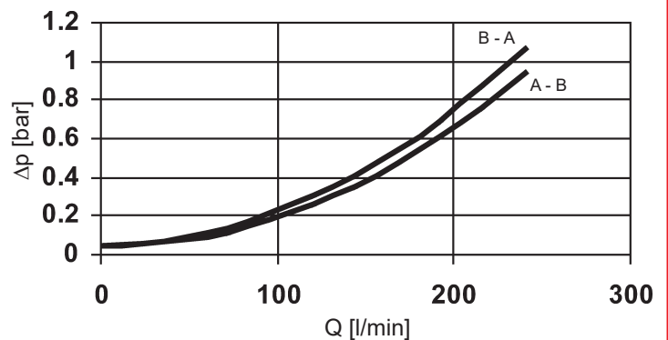
DFF 330, 500, 660, 990, 1320
