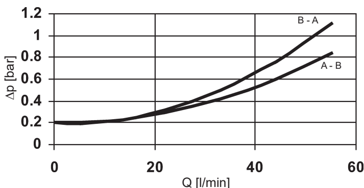
DFF 60, 110, 140
